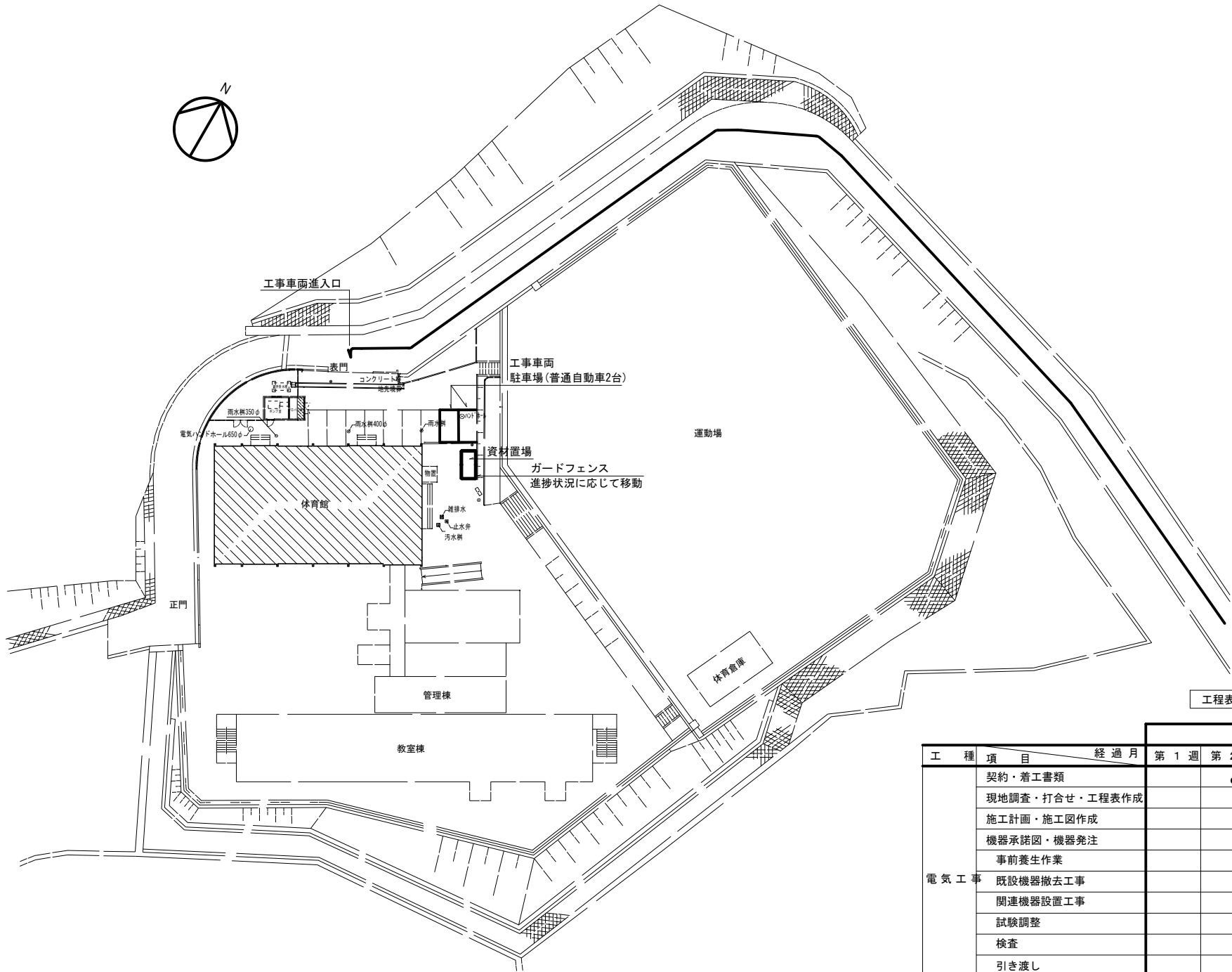
配置図 1/500
