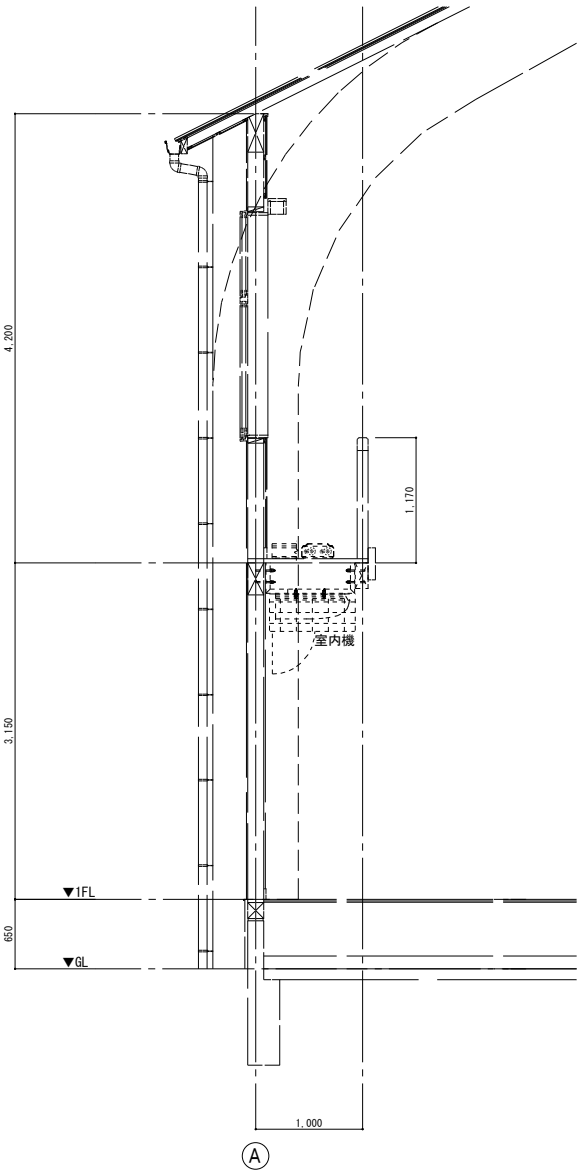
参考断面詳細図 S=1/50
